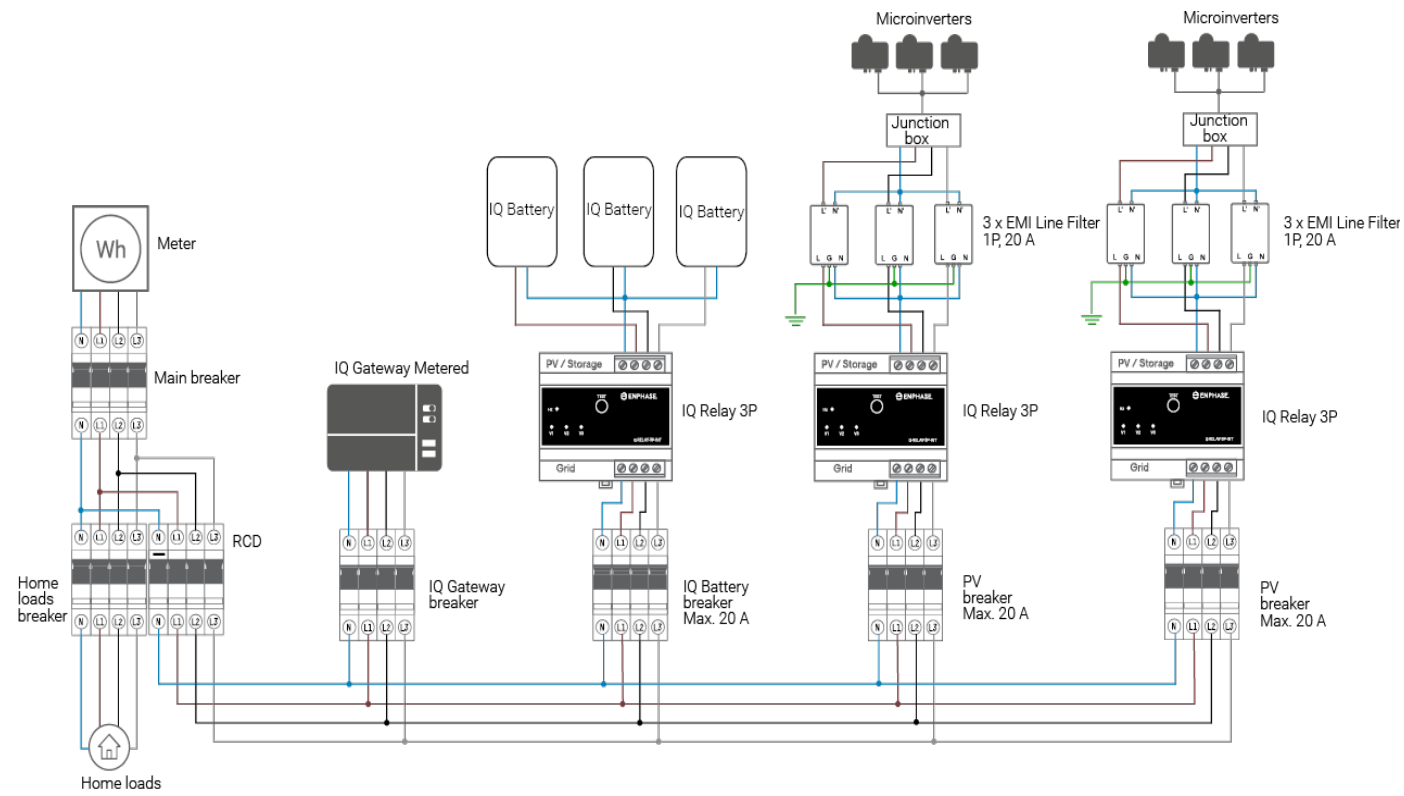
Dreiphasiges System mit mehreren Abzweigungen und Speichersystem mit EMI Line Filter
