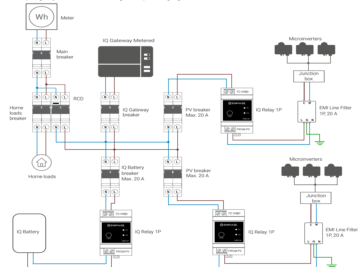
Einphasiges System mit mehreren Abzweigen und Speicherringdiagramm mit EMI Line Filter
